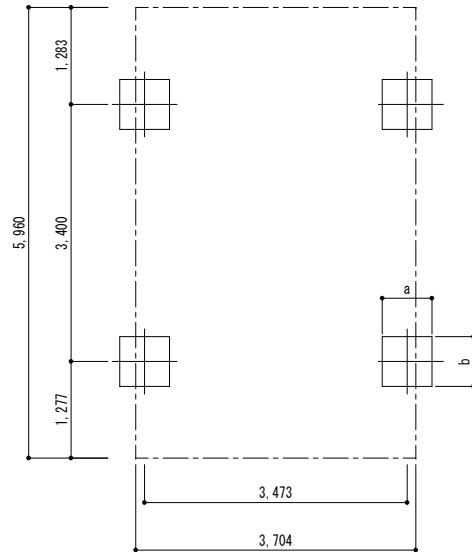
■ 基礎配置図
